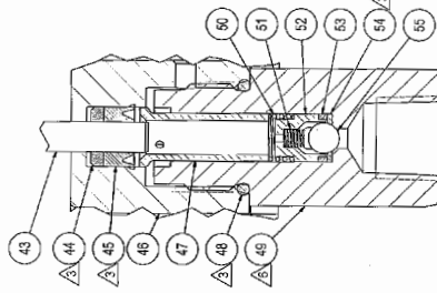
DETAIL X (MS-110)
